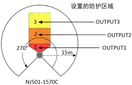
防护区域示意图2
