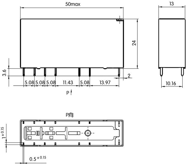
外形图
