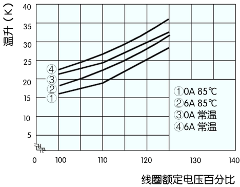
线圈温升
