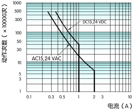
感性电耐久性曲线
