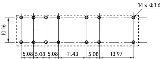
安装孔尺寸
